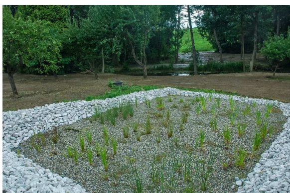
Kořenová čistírna a tůň v obci Hůrky Zdroj: https://www.korenova-cisticka.cz/
